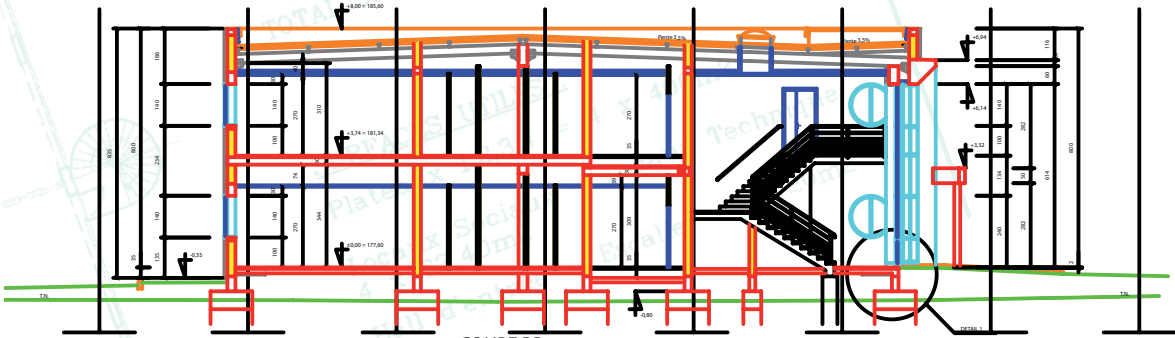
- COUPE BB -
